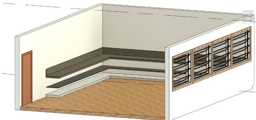
Figura 2 – Lab. de Ciências, visão 3D da bancada, prateleira em Ardósia e base com revestimento.
